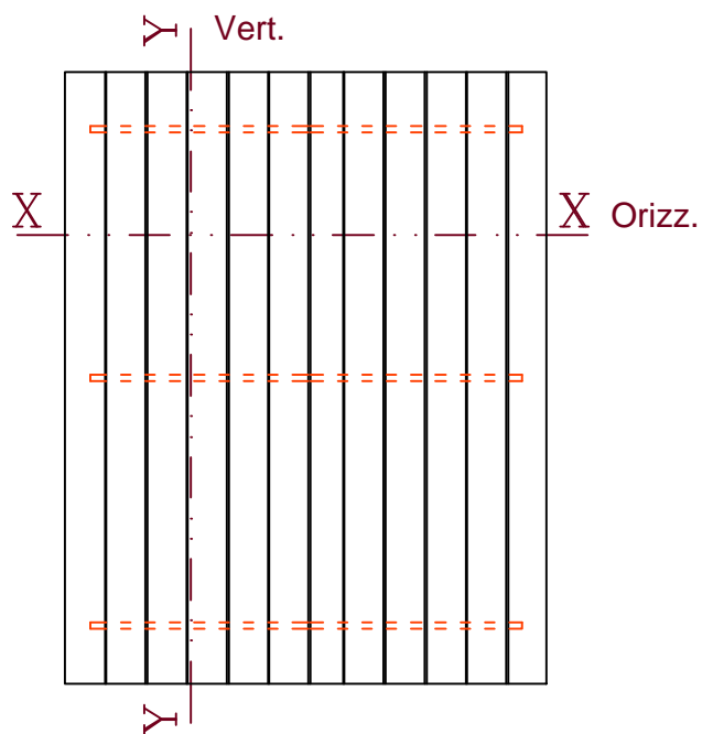
Prospetto esterno
