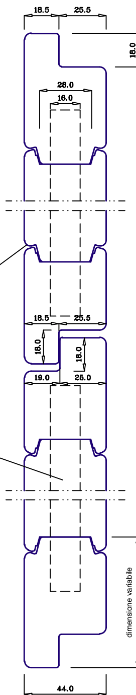
Sezione orizzontale X-X
