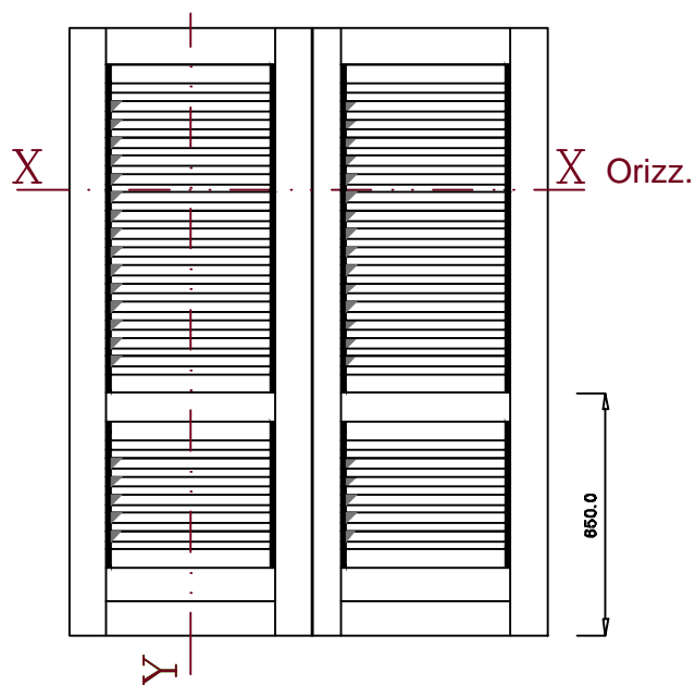
Prospetto esterno
