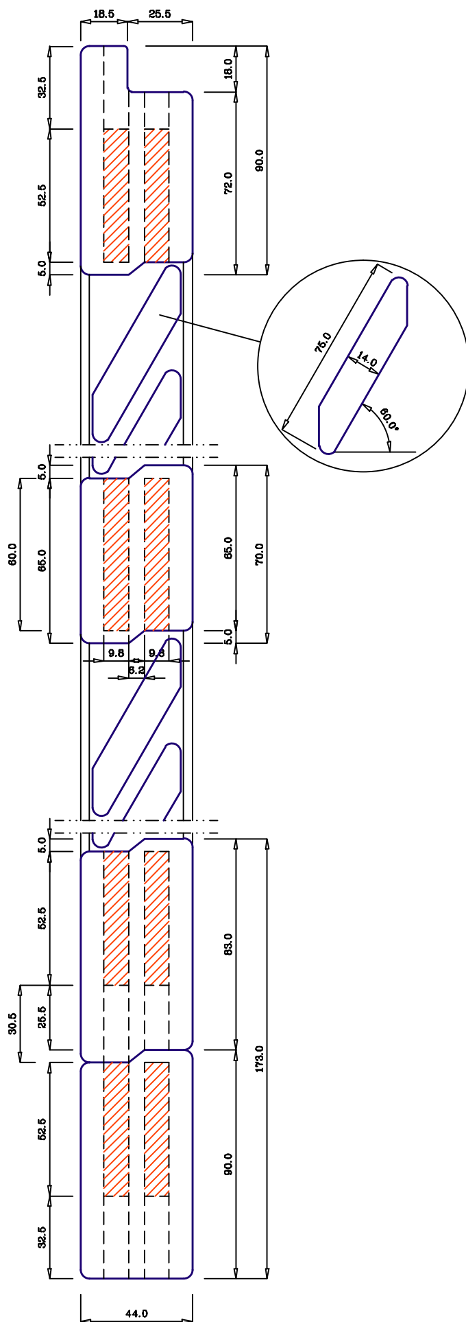
Sezione verticale Y-Y
