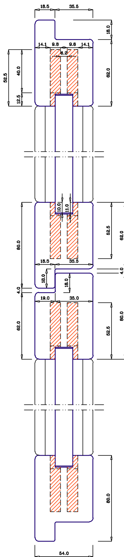
Sezione orizzontale X-X
