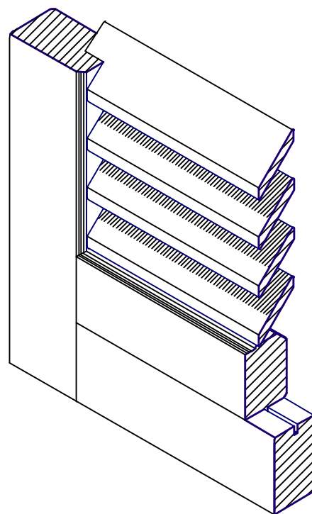
Spaccato assonometrico
