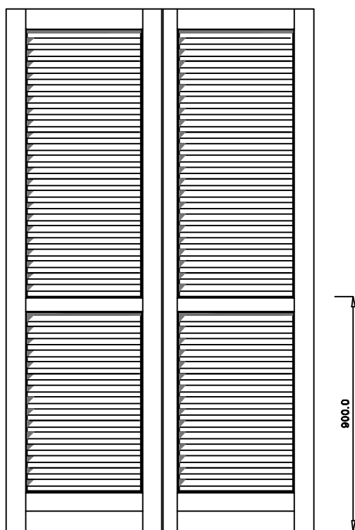
Prospetto esterno
