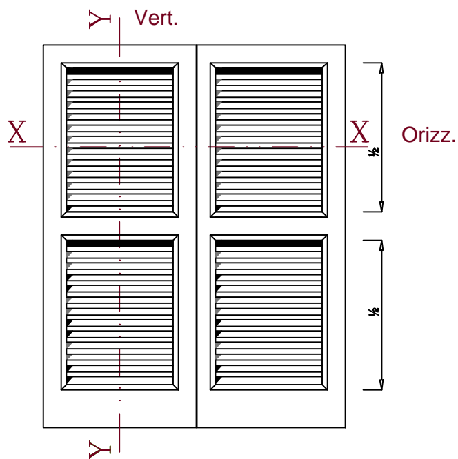
Prospetto esterno
