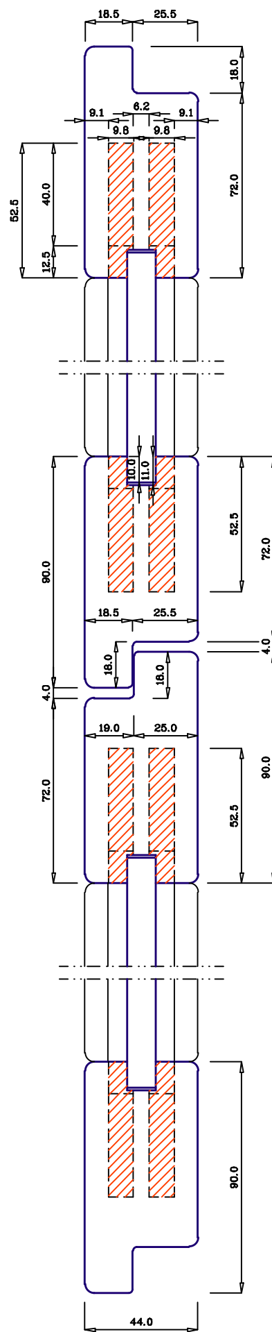
Sezione orizzontale X-X
