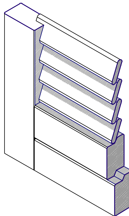
Spaccato assonometrico
