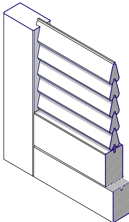
Spaccato assonometrico
