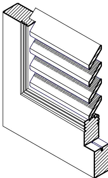
Spaccato assonometrico
