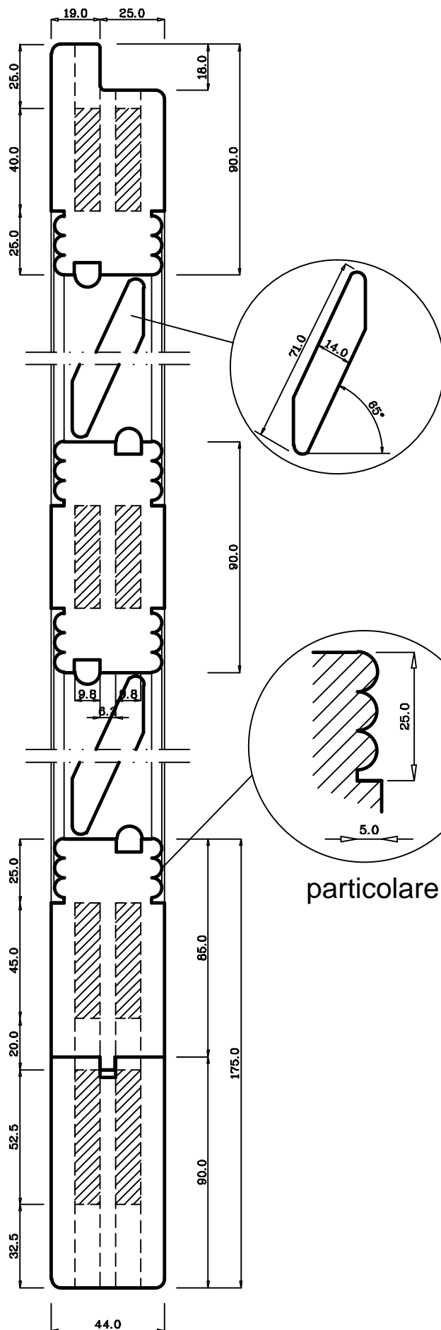
Sezione verticale Y-Y
