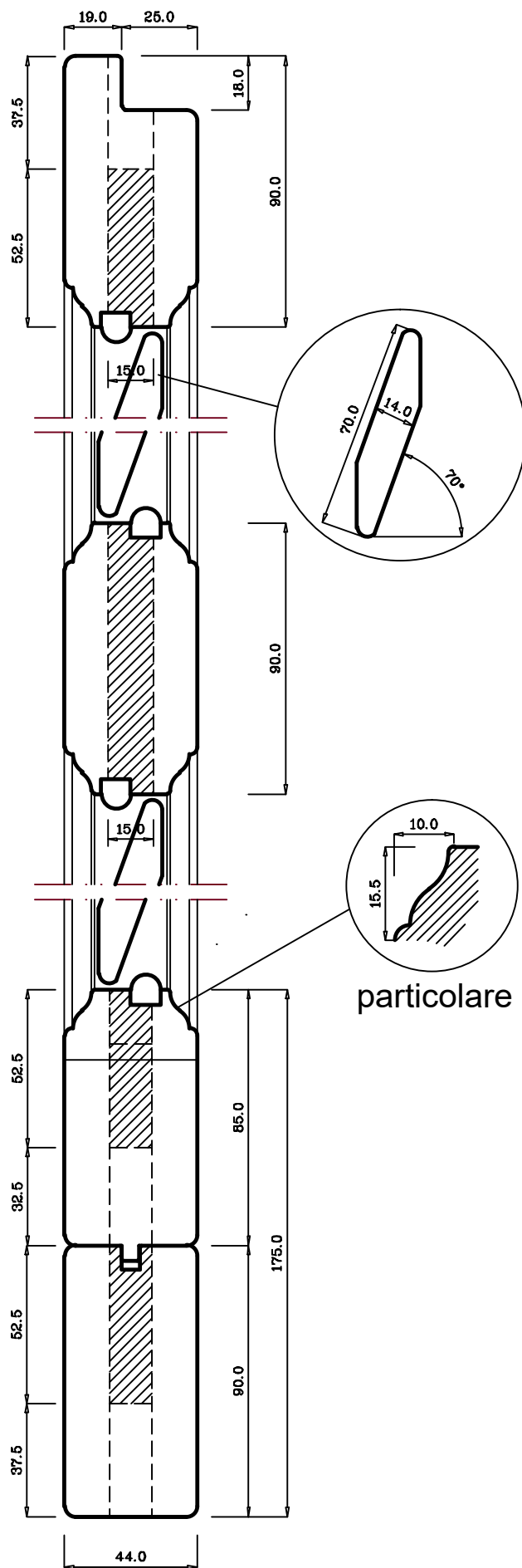
Sezione verticale Y-Y
