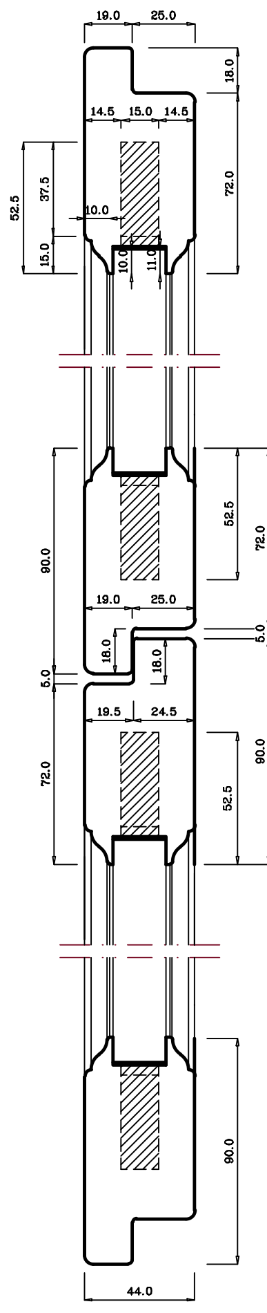
Sezione orizzontale X-X
