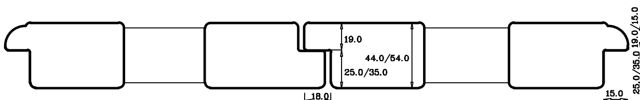
Battute 3 o 4 lati con profilo esterno sagomato
