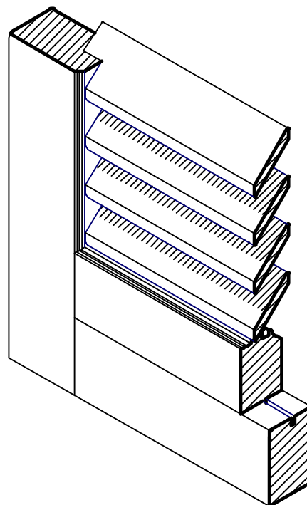
Spaccato assonometrico
