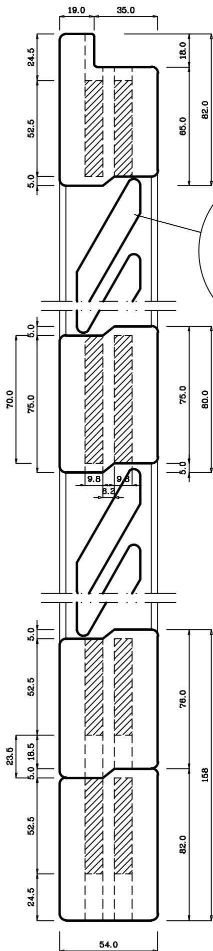
Sezione verticale Y-Y
