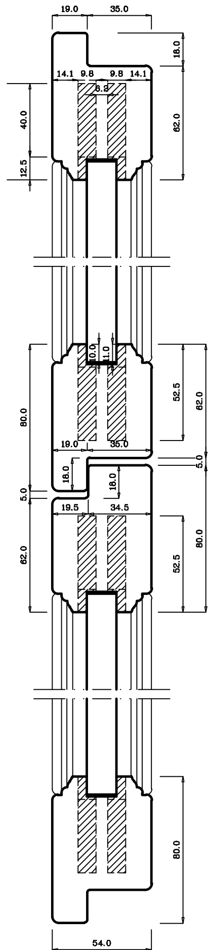
Sezione orizzontale X-X
