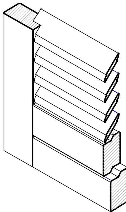
Spaccato assonometrico
