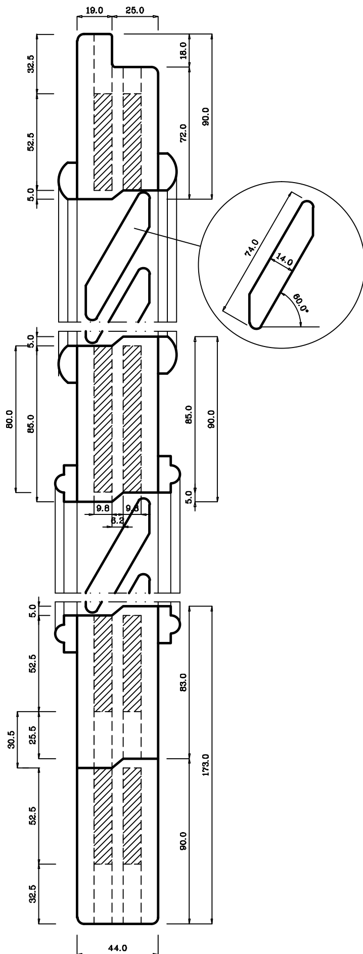
Sezione verticale Y-Y
