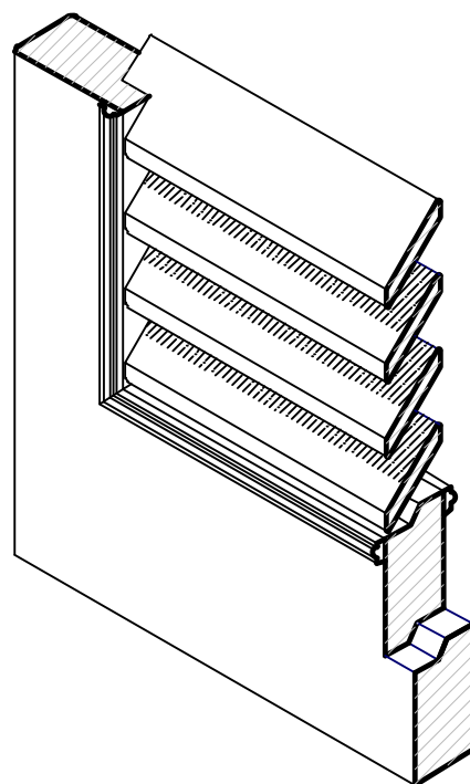
Spaccato assonometrico
