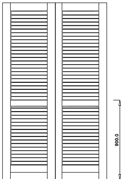
Prospetto esterno
