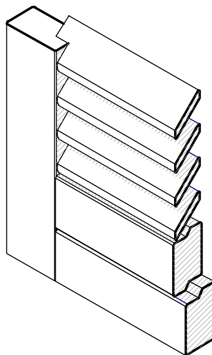
Spaccato assonometrico
