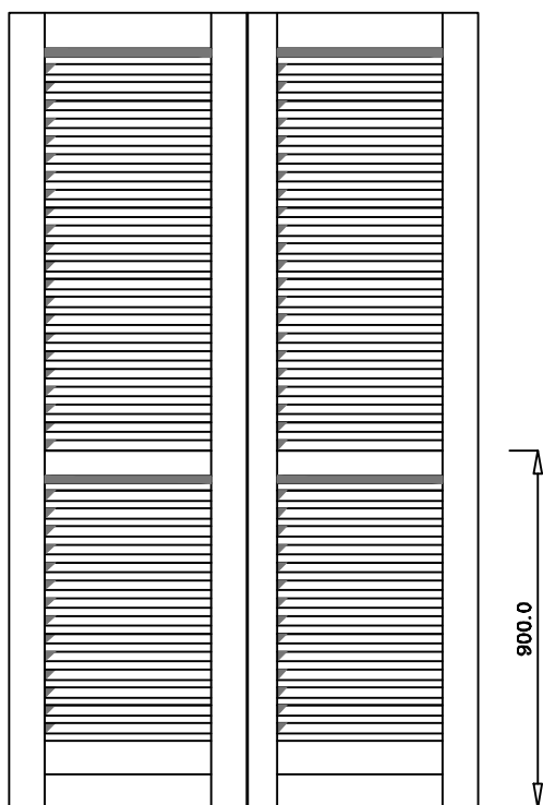
Prospetto esterno
