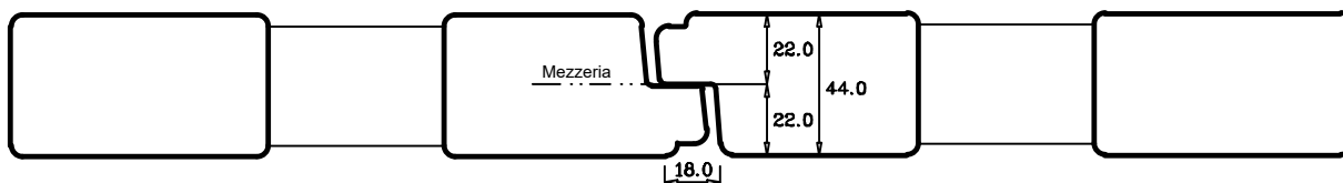
Battute al centro tipo Mako (solo sp. 44 mm.)
