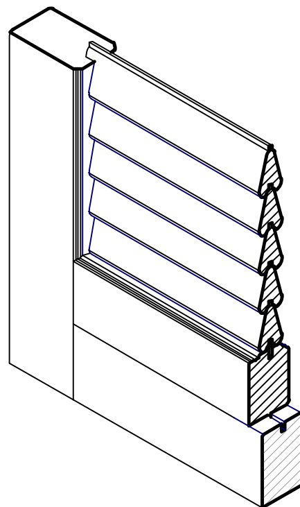
Spaccato assonometrico
