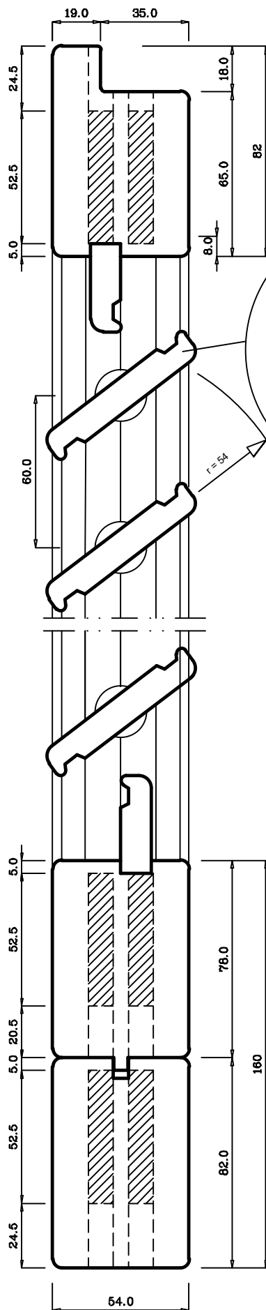
Sezione verticale Y-Y
