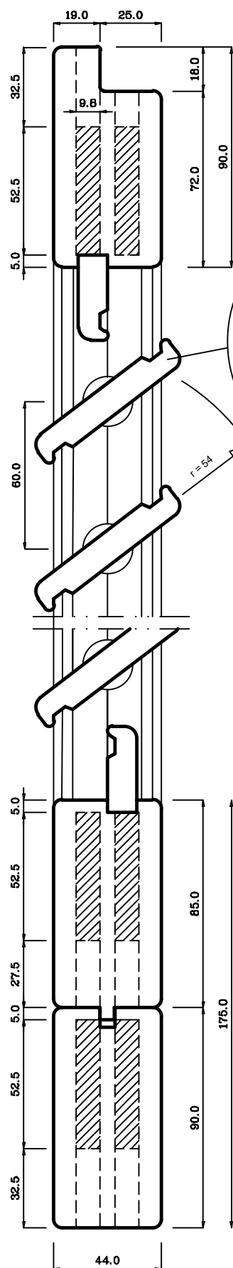
Sezione verticale Y-Y
